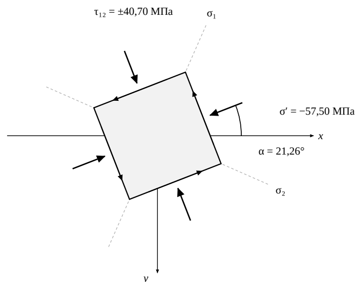
Рис. 4 — площадки с \tau_{12} = \pm 40,70 МПа в плоскости пластины. Элемент повёрнут на 45^\circ от главных направлений: \alpha = 66,26^\circ - 45^\circ = 21,26^\circ . Штриховыми показаны главные направления, на всех четырёх гранях \sigma' = -57,50 МПа.
