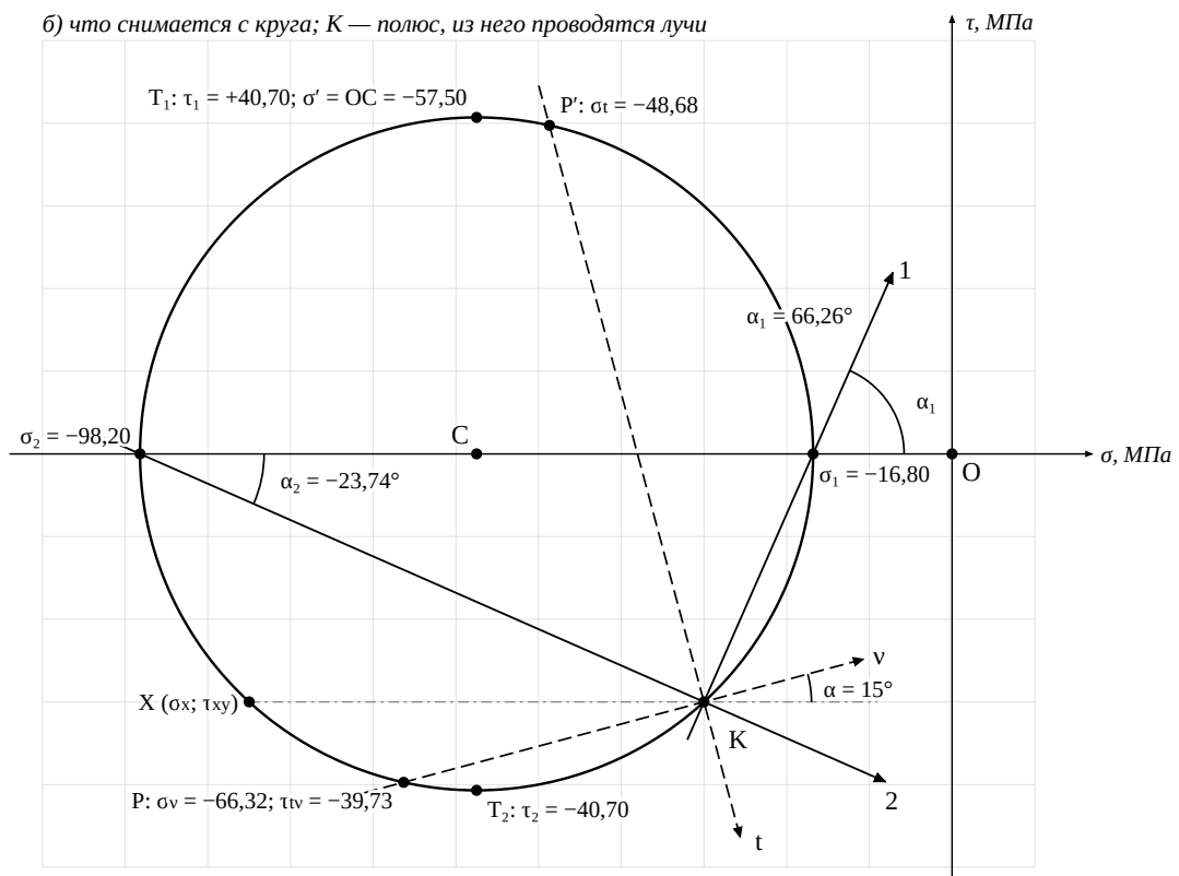
Рис. 7 — круг Мора, 1 см = 10 МПа: а) построение по \sigma_x , \sigma_y , \tau_{xy} ; б) \sigma_1 , \sigma_2 и углы \alpha_1 , \alpha_2 по лучам из полюса K, экстремальные \tau_{12} = \pm 40,70 МПа (точки T_1 , T_2 ), площадки под \alpha = 15^\circ (точки P, P').
